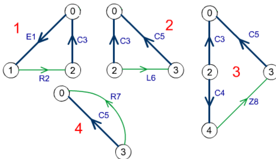
Рисунок 7. Выделение контуров.
